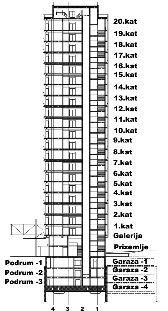
POPREČNI PRESJEK
