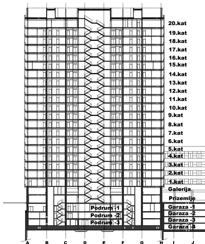
UZDUŽNI PRESJEK
