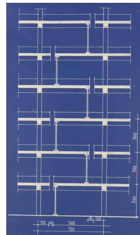
Presjek polja s privremenom dilatacijom
