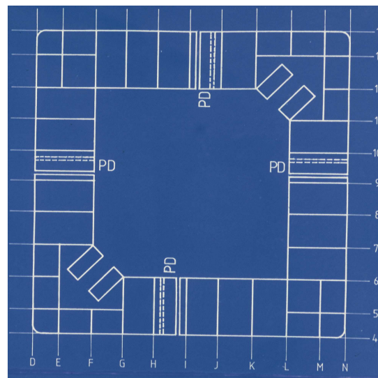
Stropna konstrukcija s položajem privremenih dilatacija
