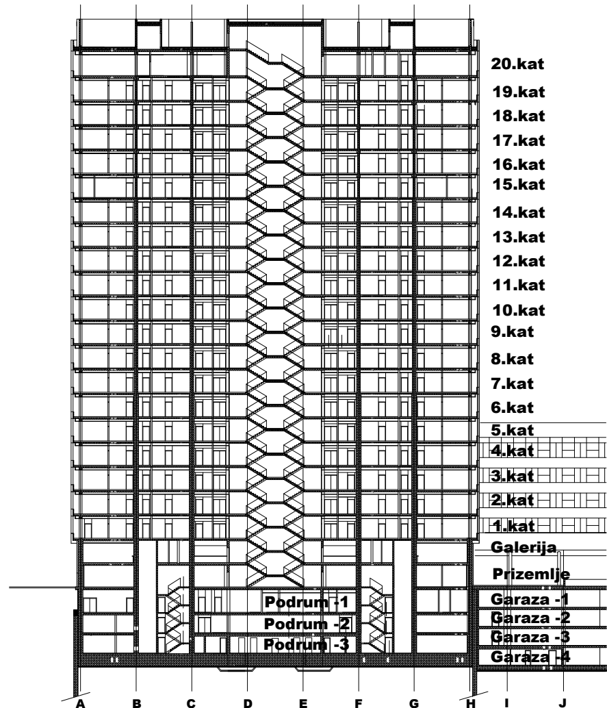
LONGITUDINAL SECTION
